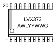
SOIC-20
