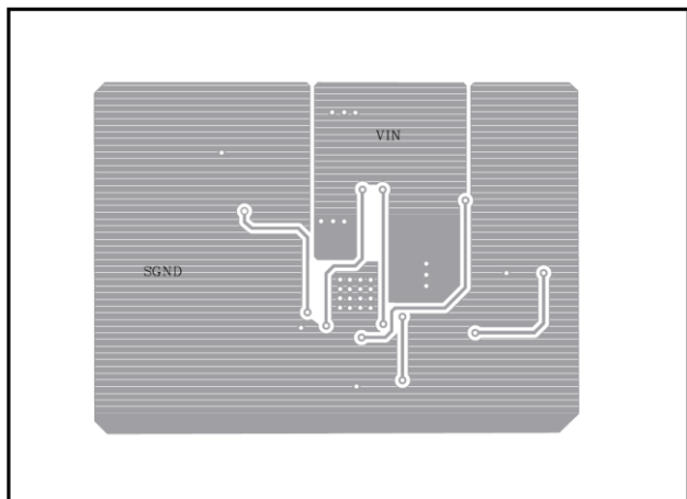
Bottom Layer
